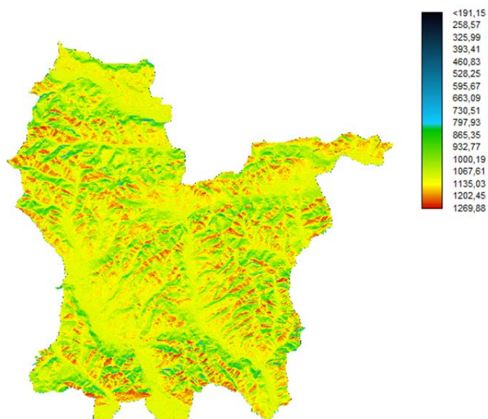
Slika 3: Globalno sončno obsevanje v Zahodnih Ljutomersko - Ormoških goricah.
